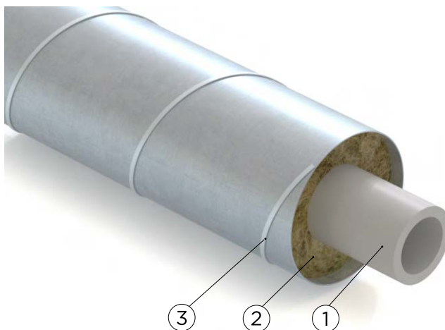
Рисунок 1.2.1. Конструкция труб СМИТФЛЕКС-П МВТ
